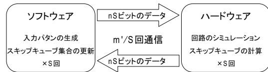
図 7 投機的実行による通信回数の削減
