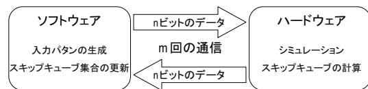
図 6 HW/SW 協調実行における通信のボトルネック
