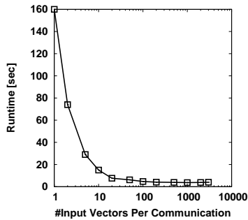
図9 検証時間の面での投機的実行の有効性 (MULT32-9の場合)
